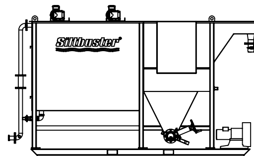
IHB10 L: 3689mm W: 1298mm H: 2387mm H: 2140mm (BRIM)
