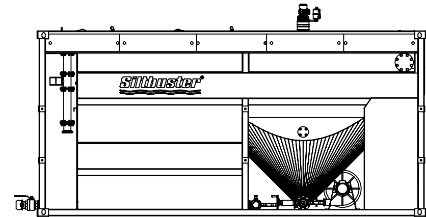
IHB40R L: 6060mm W: 2440mm H: 3303mm H: 2890mm (BRIM)
